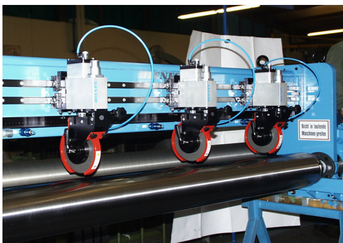
Type PQA-DF 50 1200N-8bar-1100m/min Positionnement Manuel
