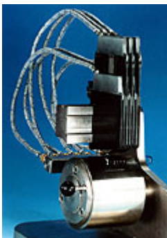
Type PQDS 6 mm 240N-6bar
